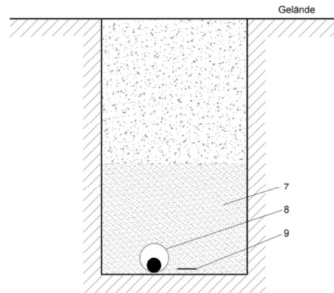
ABB. 2.2 – Verlegung des Erders bei Verwendung von Kabelschutzrohren
