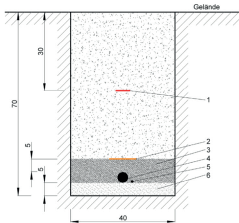
ABB. 2.1 – Erdverlegung des Erders im Nahbereich der Kabel-/Leitungsanlage
